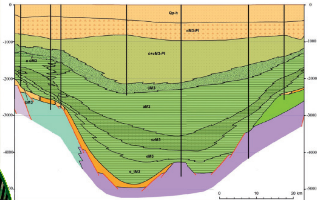
Secțiune geologică în regiunea localității Békéscsaba (modificat pe baza MÁFI, 2005): continuând de la maro către verde, bazinul adânc ce se află sub localitatea Békéscsaba este plin de roci din ce în ce mai vechi, culoarea mov ilustrează substratul mai vechi decât Miocenul. Liniile verticale negre reprezintă locurile forajelor de adâncime
