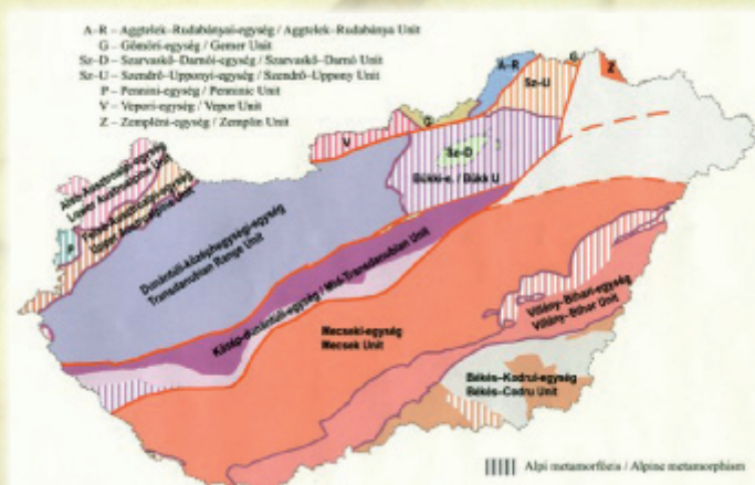
Structura subsolului din Ungaria (Haas et al. 2010)
