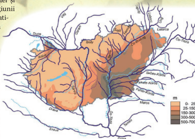
Rețeaua hidrografică a Bazinului Carpatic în Pletocenul târziu (Borsy 1989 și Gábris–Nádor 2007)
